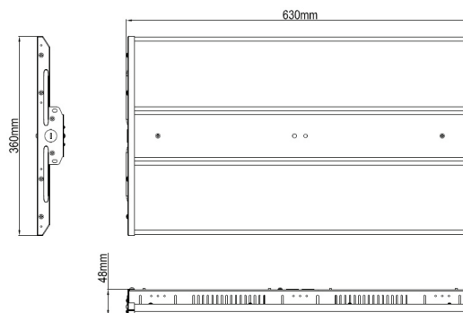
220W Dimensions
