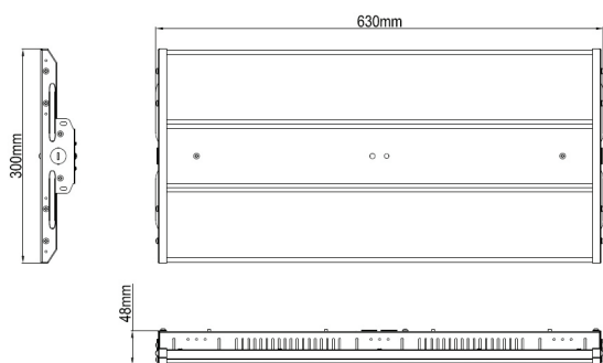
110W & 165W Dimensions
