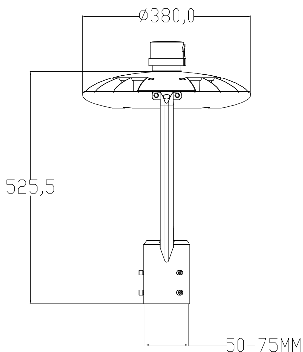
35W & 55W dimensions
